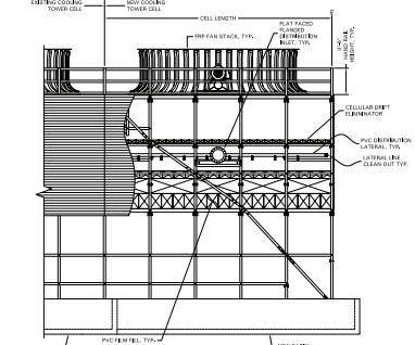
LONGITUDINAL ELEVATION
